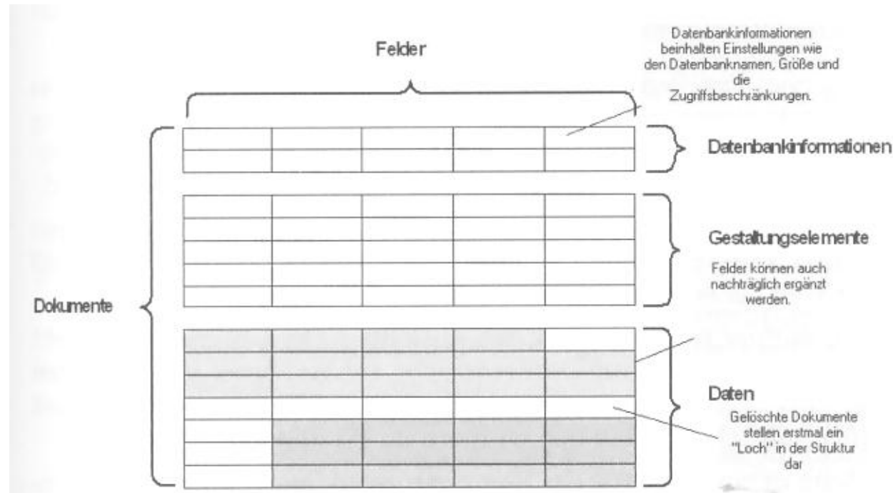
Abbildung 3.1 Aufbau einer Domino-Datenbank
